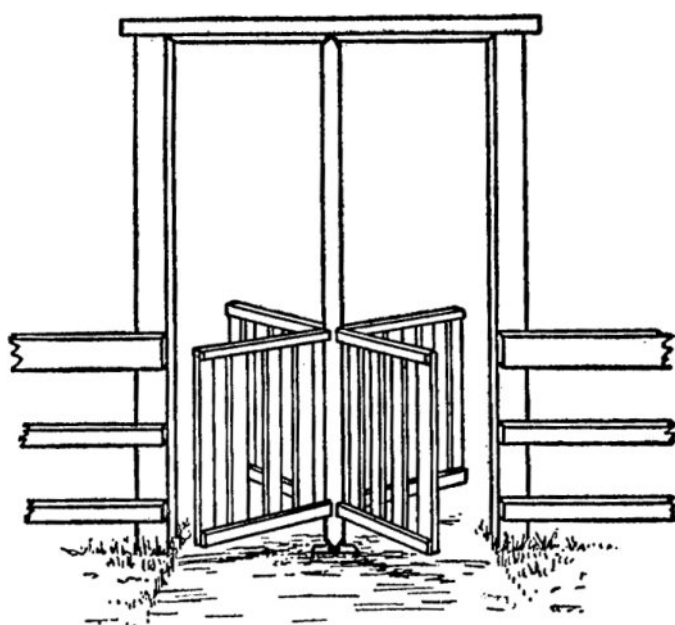
POARTĂ ROTITOARE
